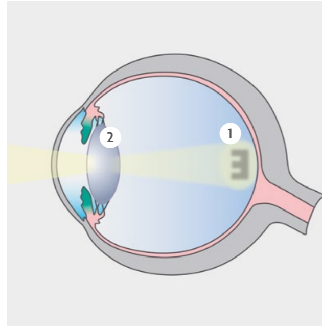
Abnahme der Sehschärfe (1) durch trübe Augenlinse (2)
